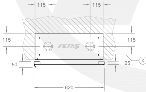
ÜST GÖRÜNÜŞ TOP VIEW
