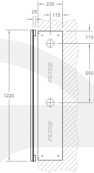
YAN GÖRÜNÜŞ SIDE VIEW
