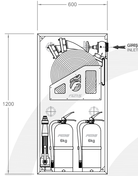
ÖN GÖRÜNÜŞ FRONT VIEW
