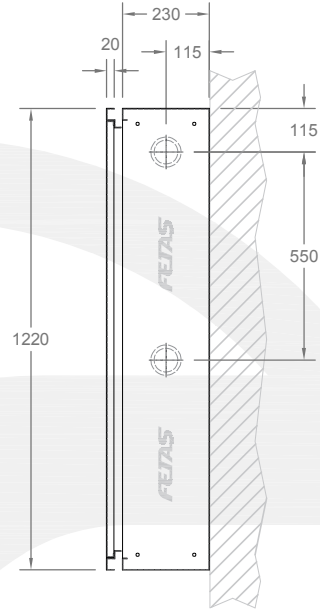
YAN GÖRÜNÜŞ SIDE VIEW
