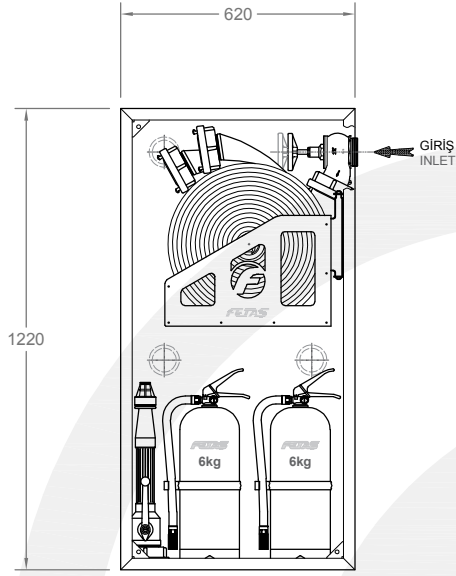
ÖN GÖRÜNÜŞ FRONT VIEW
