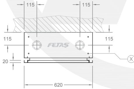
ÜST GÖRÜNÜŞ TOP VIEW
